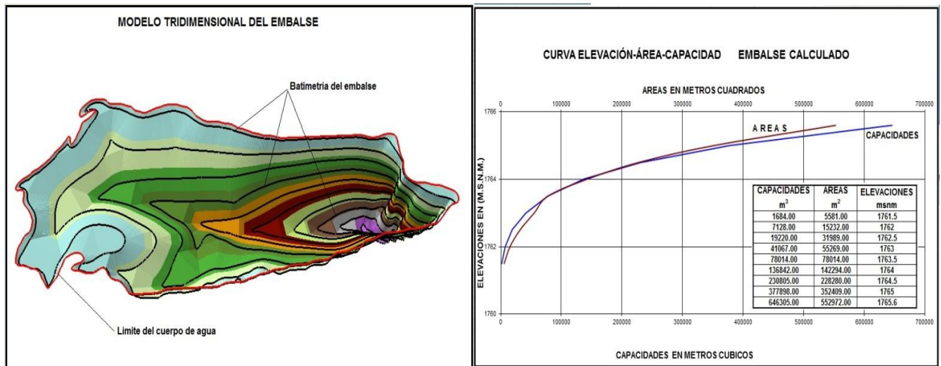
Figura 7.7. Modelo tridimensional y curva área-capacidad-elevación.
